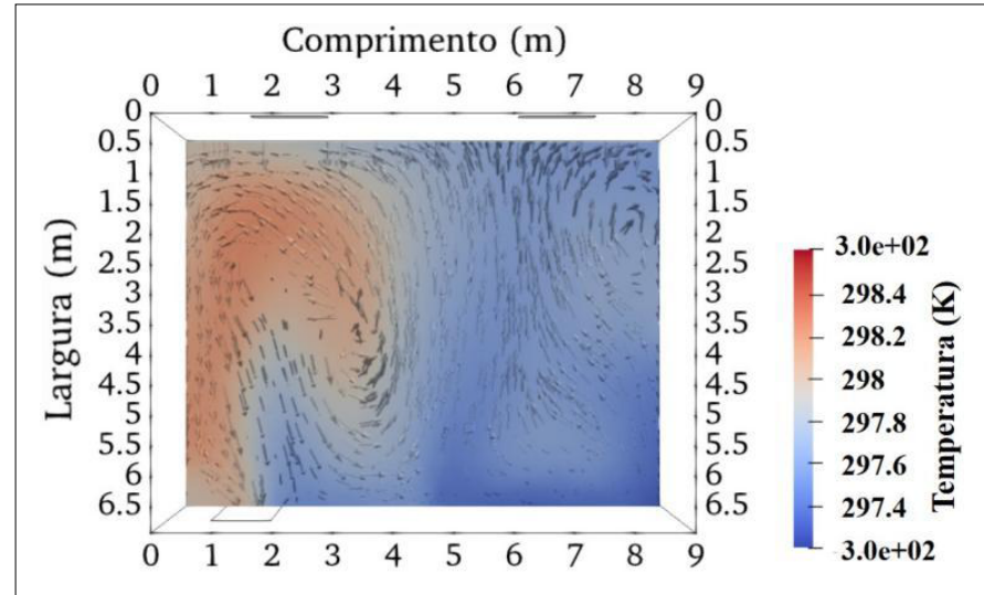
Figura 7 ► Campo vetorial de temperatura na iteração 900. Fonte: dados da pesquisa
