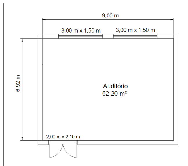
Figura 1 ► Dimensões do auditório climatizado. Fonte: elaborado pelos autores
