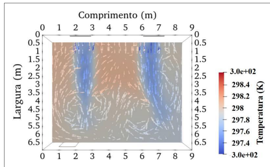
Figura 8 ► Distribuição de temperatura na região de insuflamento. Fonte: dados da pesquisa
