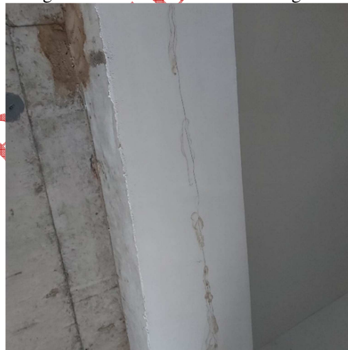
Figura 9 – Evidência de trincas no gesso
