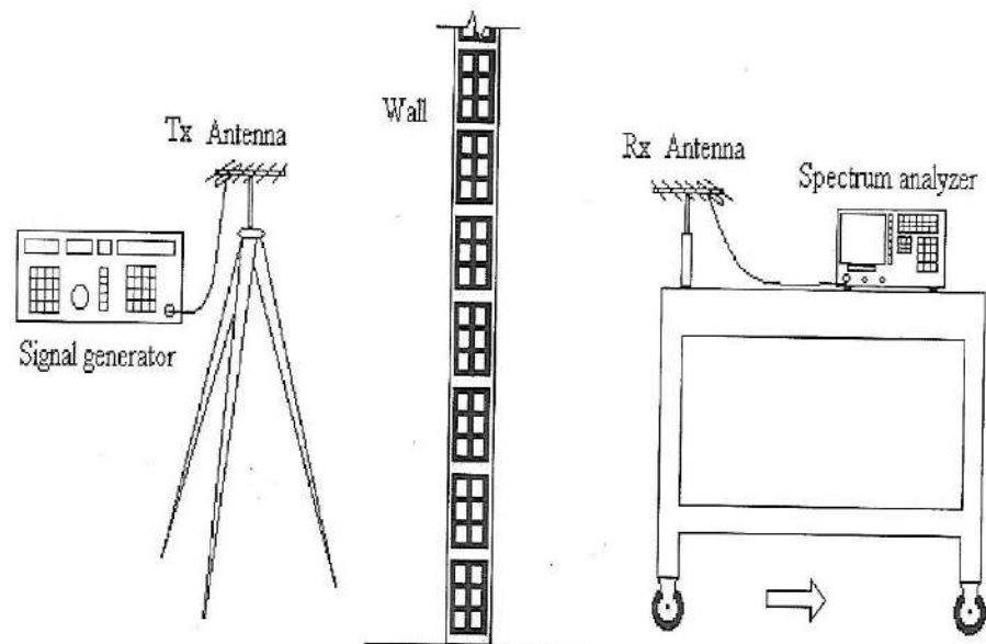
Fig. 1. Set-up de medição
