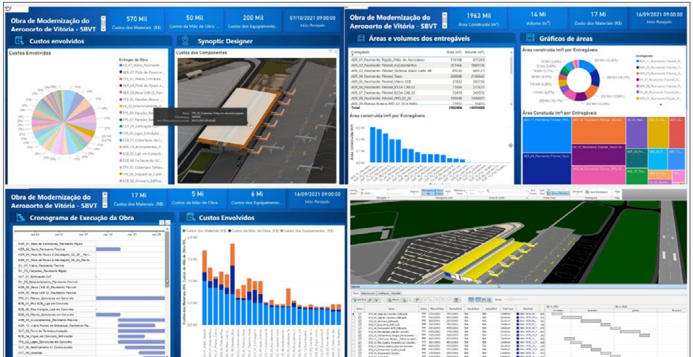
Figura 16 ▼ Exemplo do uso do Power BI integrado ao modelo BIM. Fonte: arquivo dos autores
