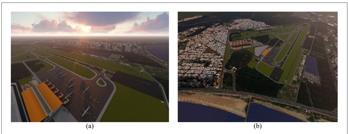
Figura 7 ▼ Modelo BIM do complexo aeroportuário. Fonte: arquivo dos autores
