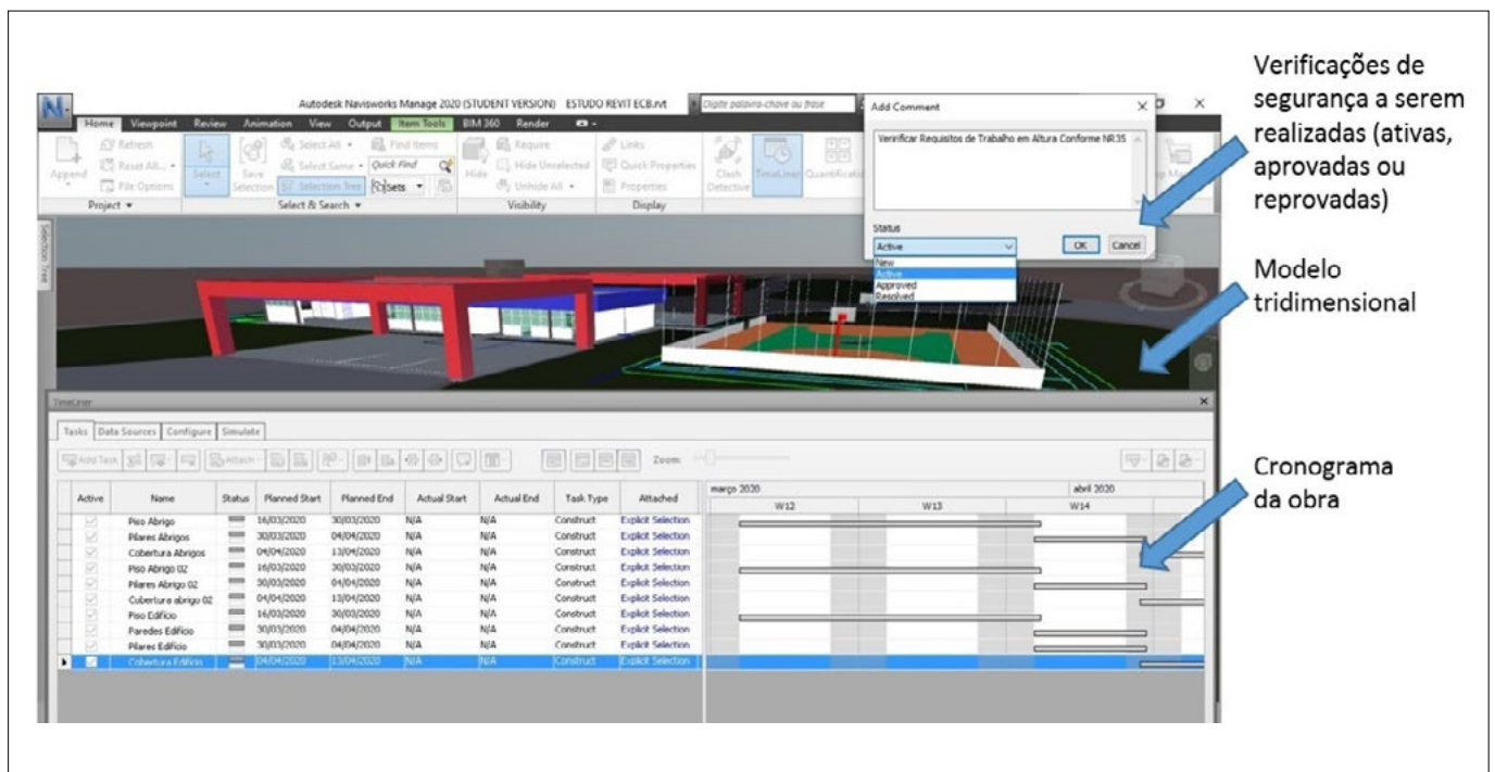
Figura 8 ▼ Agrupamento de procedimentos de segurança ao modelo BIM e ao cronograma físico da obra. Fonte: arquivo dos autores
