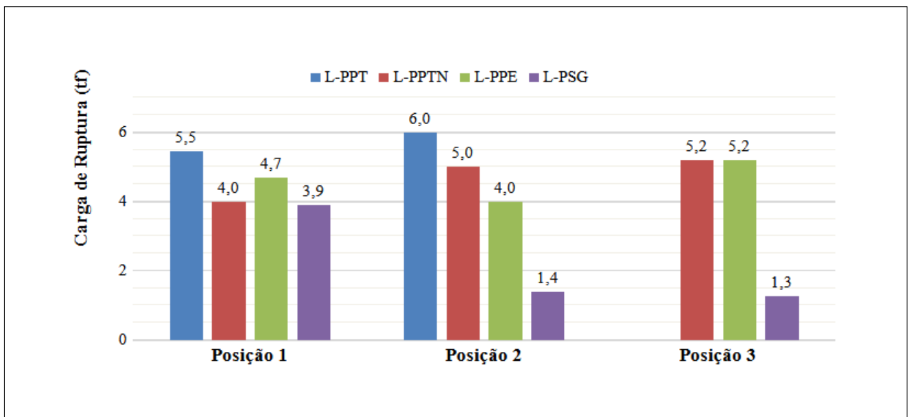
Figura 6 ▼ Cargas de ruptura dos sistemas. Fonte: dados da pesquisa (2019)
