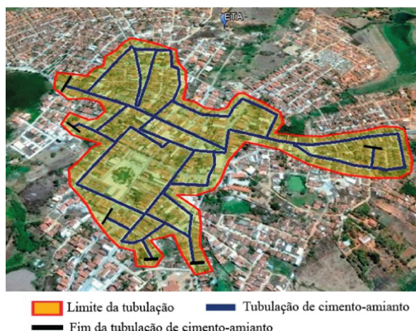
Figura 6. Mapeamento digital da tubulação em estudo.
