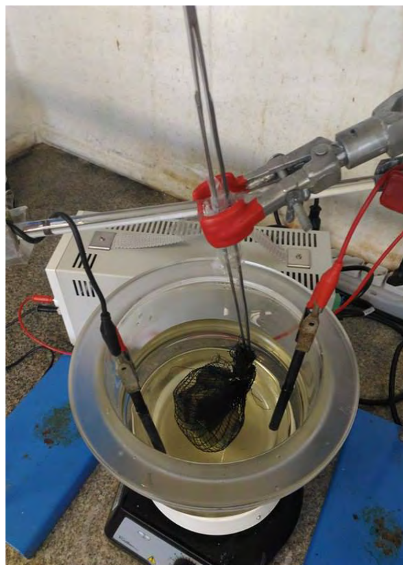
Figura 2 – Escala de bancada do processo de eletrorremoção
