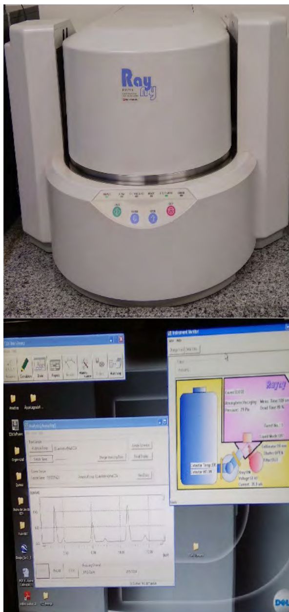
Figura 1 – Espectrofotômetro de energia dispersiva de raios-x, marco Shimatzu modelo 700-MS, utilizado nas medições de concentrações dos metais
