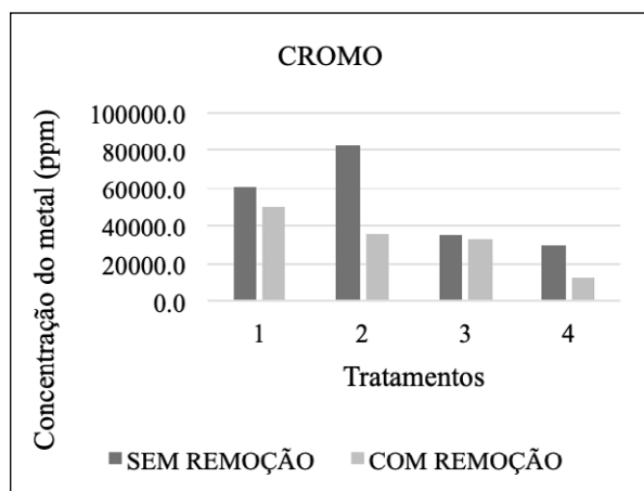
Figura 4 – Distribuição do metal cromo nos diferentes tratamentos de CCA aplicados, nas concentrações de 1 a 3, de acordo com a taxa de remoção obtida
