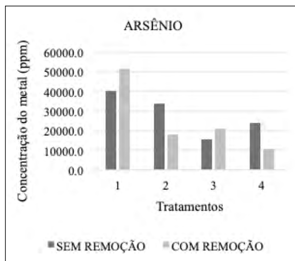
Figura 5 – Distribuição do metal de arsênio nos diferentes tratamentos de CCA aplicados, nas concentrações de 1 a 3, de acordo com a taxa de remoção obtida
