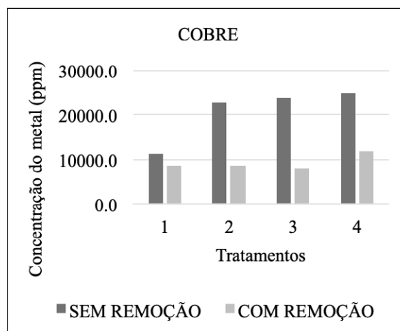
Figura 3 – Distribuição do metal de cobre nos diferentes tratamentos de CCA aplicados, nas concentrações de 1 a 3, de acordo com a taxa de remoção obtida
