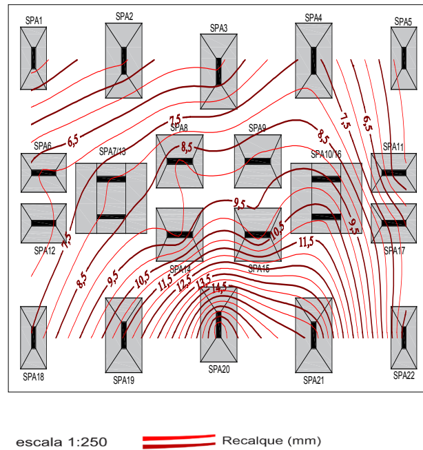
Figura 4 ▶ Curvas de isorrecalques torre "A" – Estágio 3. Fonte:Santos (2018)
