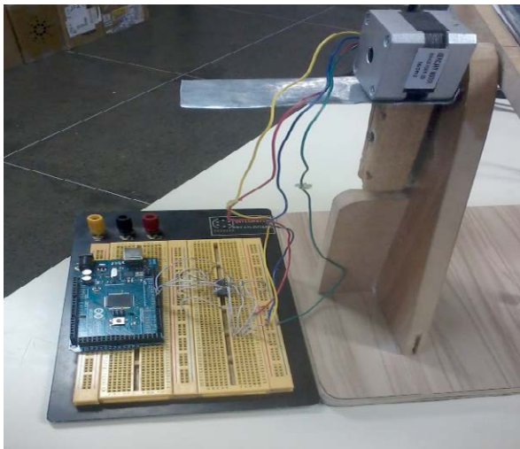
Figura 3 – Montagem do Circuito
