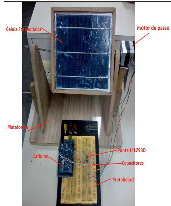
Figura 4 – Equipamento Montado
