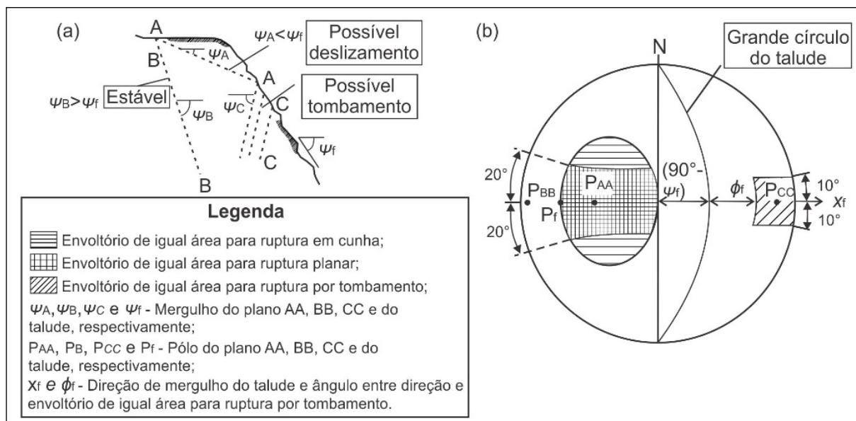
Figura 3 – Análise cinemática dos blocos de rocha no talude: (a) família de descontinuidades no talude; e (b) envoltórios de igual área em estereograma.
