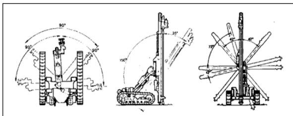
Figura 5 – Exemplo de perfuratriz com martelo de superfície sobre trator com esteiras, muito versátil quanto à mobilidade e angulação de trabalho, bastante utilizada em desmontes realizados em bancadas (principalmente em pedreiras)
