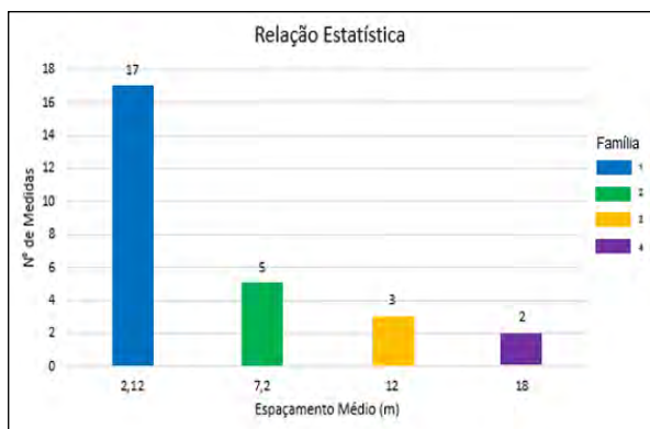
Figura 10 – Relação estatística entre o número de medidas, por família, e o espaçamento médio delas.
