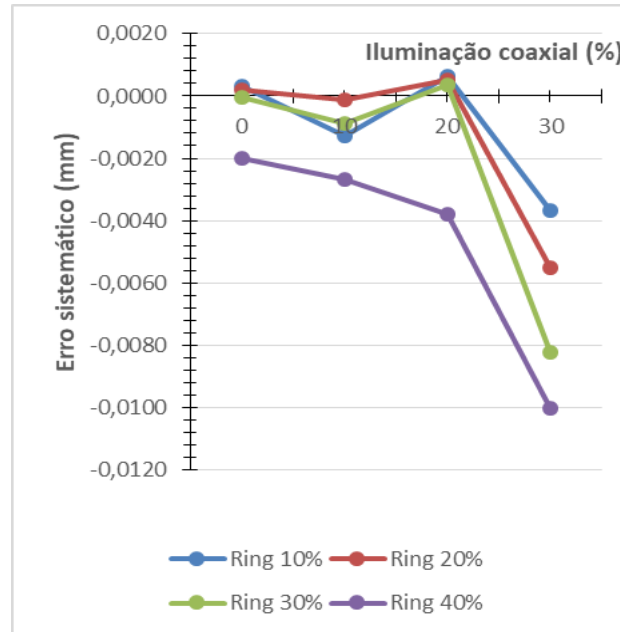
Figura 11 ► Gráfico do erro sistemático em função da iluminação coaxial. Fonte: dados da pesquisa
