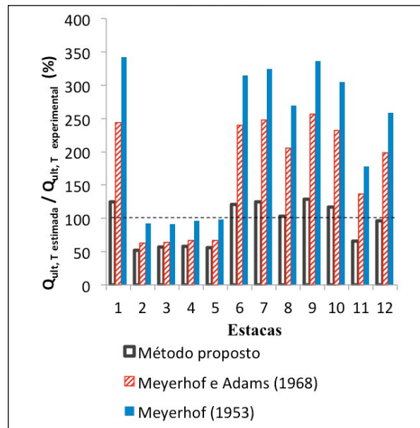
Figura 11 – Avaliação das previsões da carga última à tração a partir da equação proposta e utilizando os métodos específico e não específico mais concordantes
