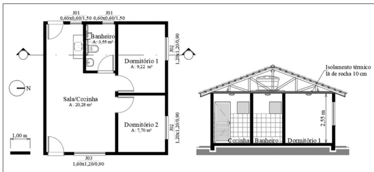
Figura 1 – Planta baixa e corte da edificação (todas as dimensões são dadas em metros)
