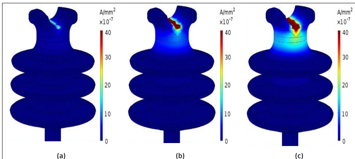
Figura 10 – Densidade de corrente no isolador 1 com poluição: (a) leve, (b) intermediária e (c) elevada
