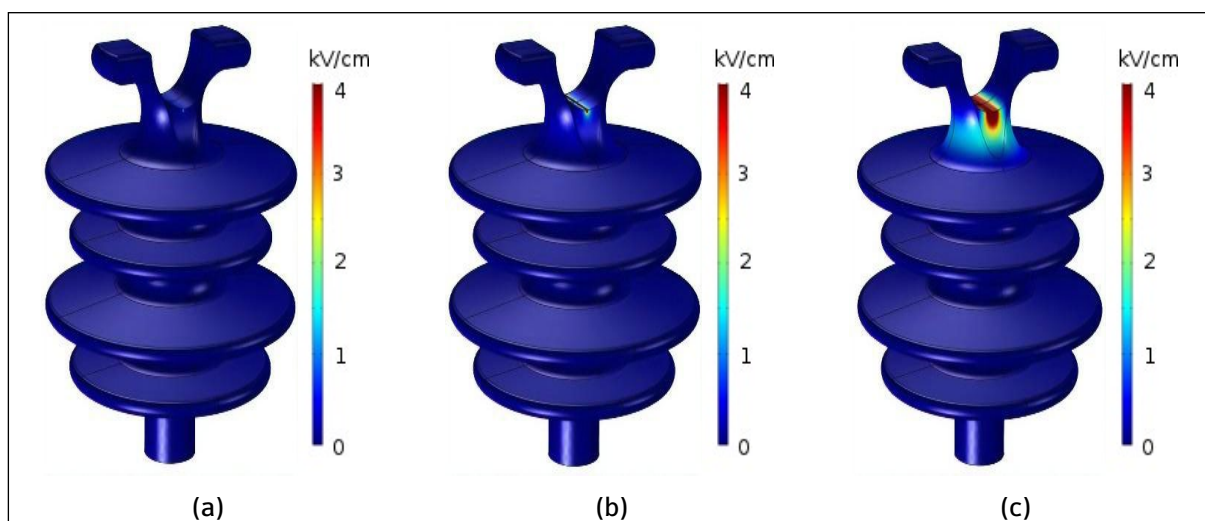
Figura 14 – Distribuição do campo elétrico no isolador 2 com poluição: (a) leve, (b) intermediária e (c) elevada
