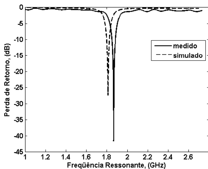
Figura 12. Perda de retorno da antena fractal de Koch de nível 1 com contornos triangulares.
