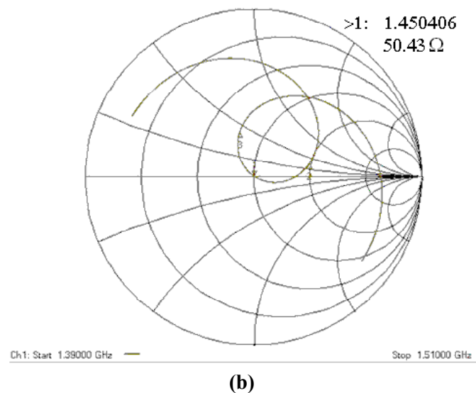
Figura 14. Cartas de Smith indicando a variação da impedância de entrada das antenas fractais de Koch de nível 2: (a) com contornos triangulares; (b) com contornos retangulares.
