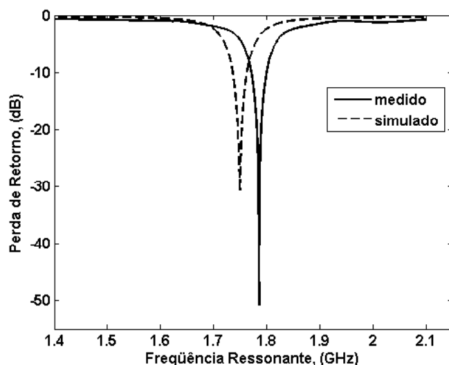
Figura 13. Perda de retorno da antena fractal de Koch de nível 2 com contornos triangulares.
