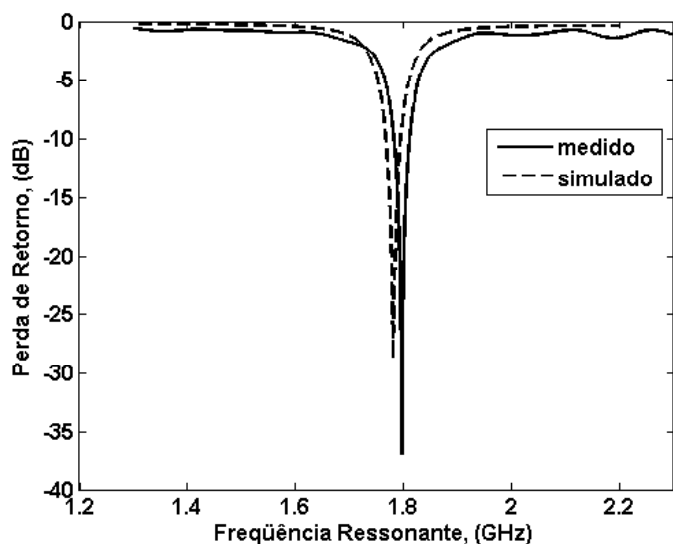
Figura 10. Perda de retorno da antena fractal de Koch de nível 1 com contornos retangulares.
