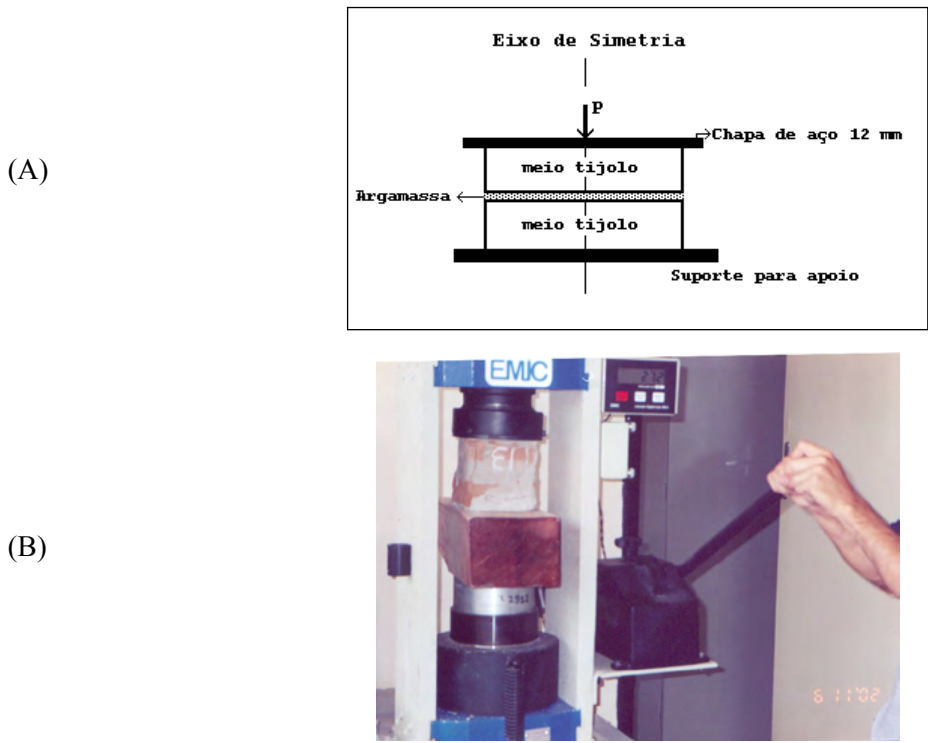
Figura 2. (A) Esquema do preparo do bloco para o ensaio de resistência à compressão simples e (B) Execução do ensaio.
