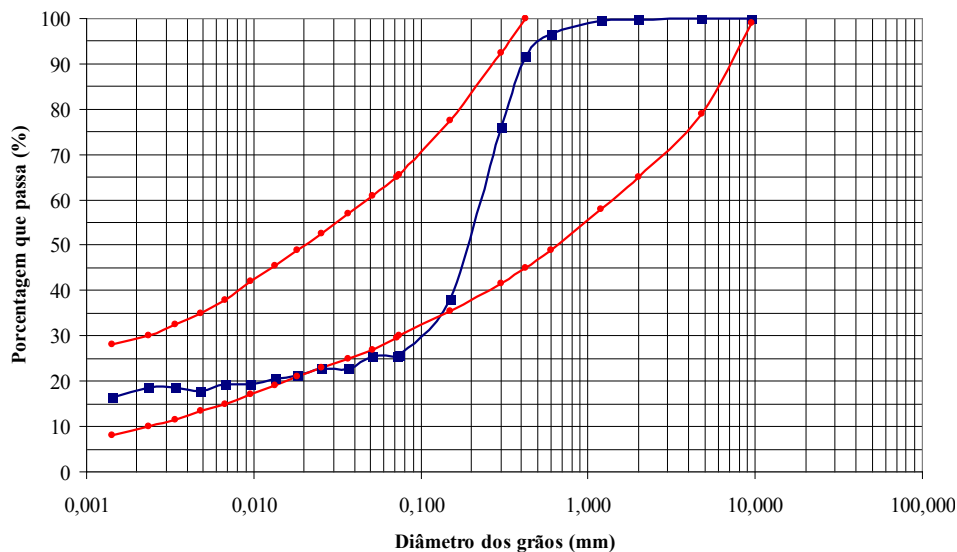
Figura 5. Curva granulométrica do solo.
