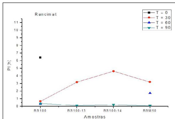
Figura 5 – Rancimat dos biodieseis metílicos de soja
