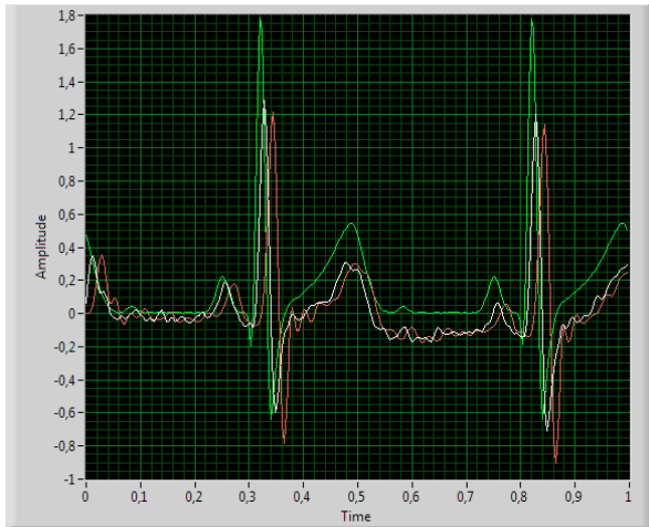
Figura 3 – Comparação entre os sinais de ECG. (a) Filtro passa-baixas Butterworth de ordem 2 e 8. (b) Filtro passa-baixas Chebyshev de ordem 2 e 8.
