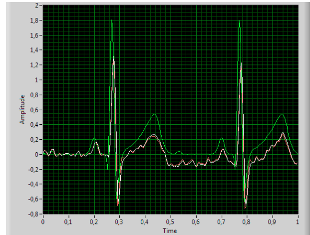
Figura 5 – Análise do sinal de ECG com filtro passa-baixas Butterworth de ordem 2, para diferentes frequências de corte.
