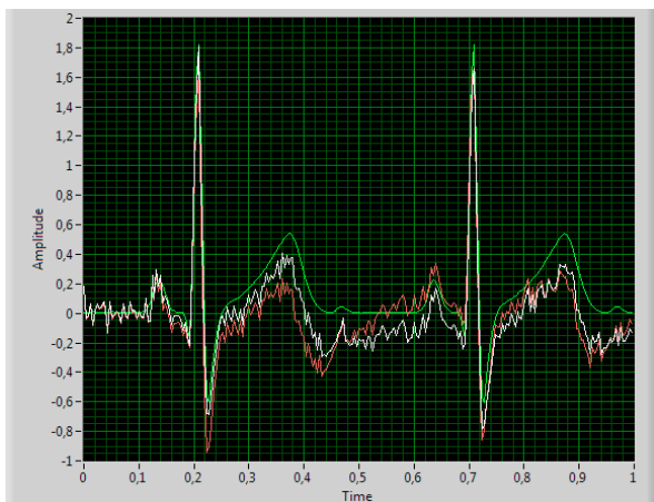
Figura 7 – Comparação entre os sinais de ECG, após os filtros passa-altas Butterworth de ordem 2 e 8.
