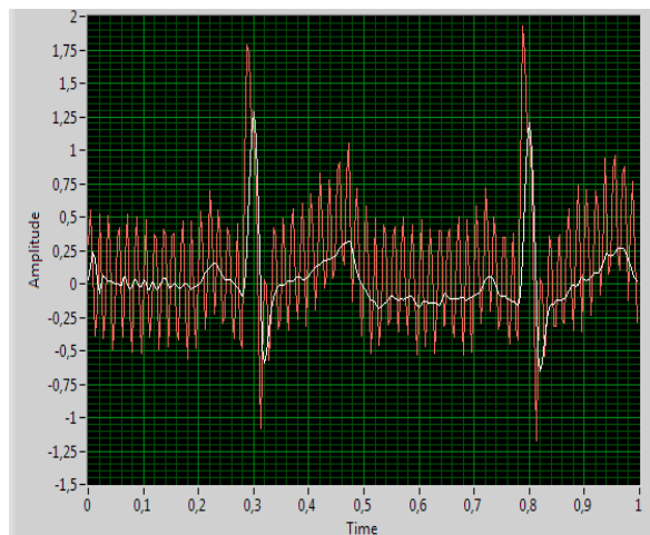
Figura 8 – Sinais de ECG. (a) Com acréscimo de ruído e após a etapa de filtragem. (b) Sem acréscimo de ruído e após a etapa de filtragem.
