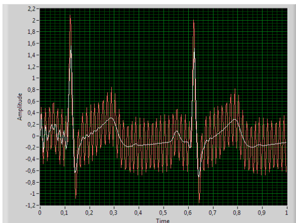
Figura 7 – Comparação entre os sinais de ECG, após os filtros passa-altas Butterworth de ordem 2 e 8.
