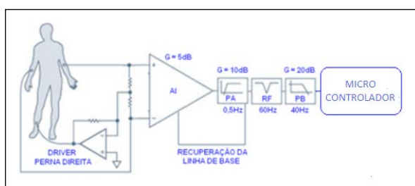
Figura 1 – Modelo de um condicionamento de um sinal ECG.
