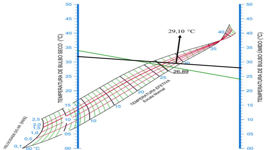
Figura 1 – Nomograma para determinação da temperatura efetiva (TE) em função da temperatura de bulbo seco, bulbo úmido e velocidade do ar. Fonte: adaptado de ELEFANT 6 , sem data.
