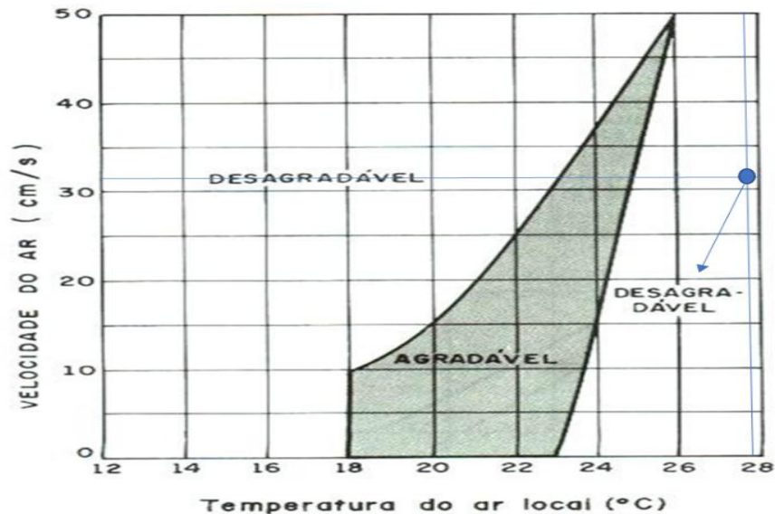
Figura 2 – Região de conforto em função da temperatura local e velocidade do ar. Fonte: adaptado de MACYNTIRE 7 , 2008.
