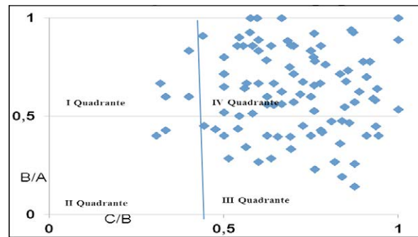
Figura 4 – Classificação das formas de agregados, relação de C/B e B/A
